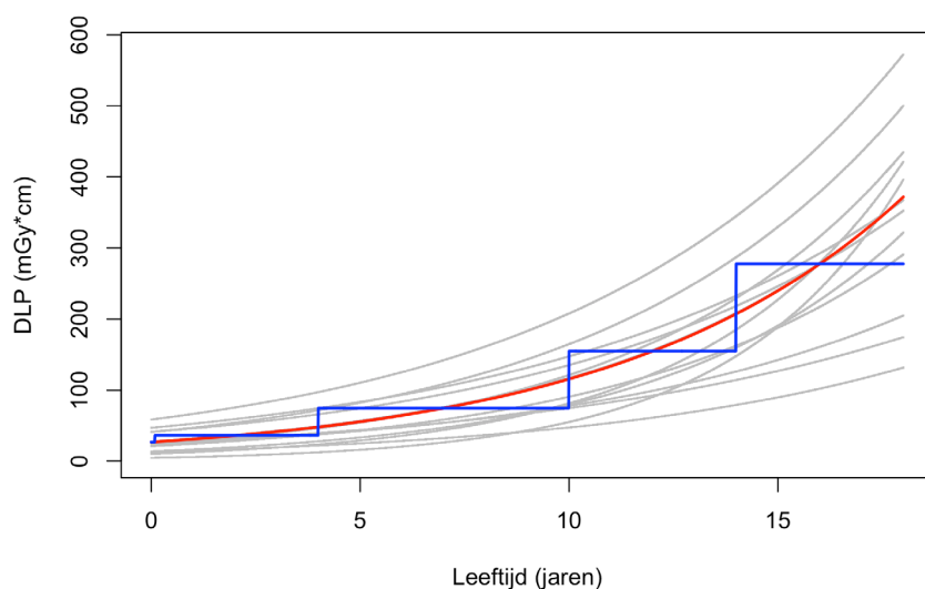
Figuur S2.8 – Vastgestelde DRN CT abdomen – DLP(leeftijd) = 26,8 \times e^{(0,15 \times leeftijd)} Gebaseerd op data van 18 centra. Rode lijn: vastgestelde DRN (75 e percentiel) Blauwe lijn: DRN per leeftijdscategorie Grijs lijnen: individuele centra.
