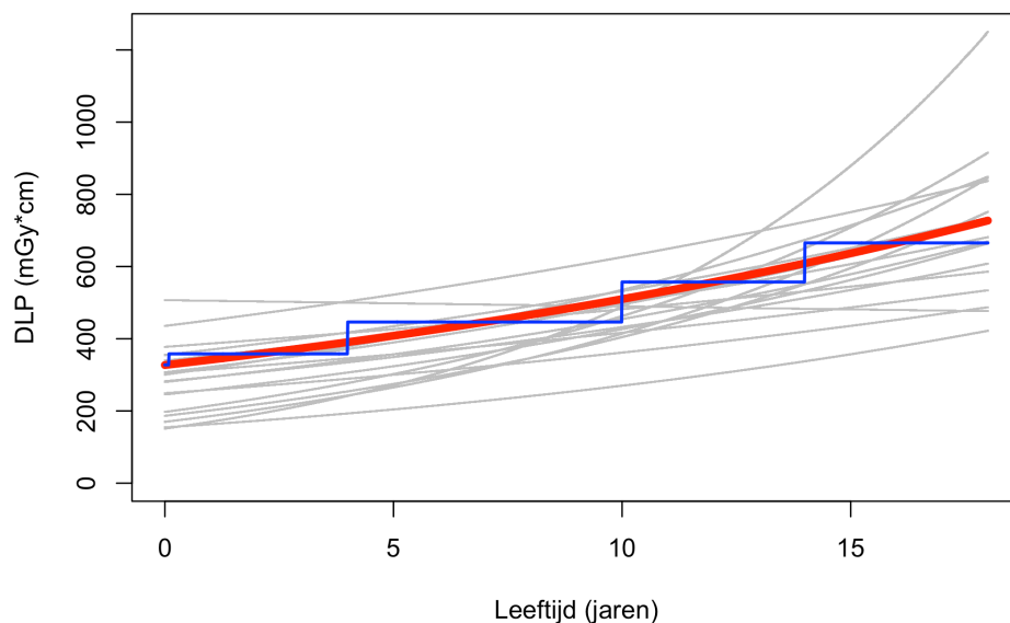
Figuur S2.5 – Vastgestelde DRN CT hersenen - DLP(leeftijd) = 327,0 \times e^{(0,04 \times leeftijd)}
