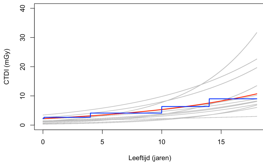
Figuur S2.2 – Vastgestelde DRN CT CWK - CTDI_{vol}(leeftijd) = 2,2 \times e^{(0,09 \times leeftijd)} Gebaseerd op data van 12 centra. Rode lijn: vastgestelde DRN (75 e percentiel) Blauwe lijn: DRN per leeftijdscategorie Grijs lijnen: individuele centra.
