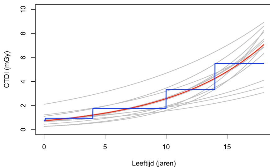
Figuur S2.4 – Vastgestelde DRN CT abdomen- CTDI_{vol}(\text{leeftijd}) = 0,7 \times e^{(0,13 \times \text{leeftijd})} Gebaseerd op data van 18 centra. Rode lijn: vastgestelde DRN (75 e percentiel) Blauwe lijn: DRN per leeftijdscategorie Grijs lijnen: individuele centra.
