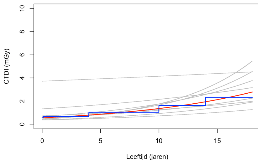
Figuur S2.3 – Vastgestelde DRN CT thorax - CTDI_{vol}(\text{leeftijd}) = 0,6 \times e^{(0,09 \times \text{leeftijd})} Gebaseerd op data van 11 centra. Rode lijn: vastgestelde DRN (75 e percentiel) Blauwe lijn: DRN per leeftijdscategorie Grijs lijnen: individuele centra.
